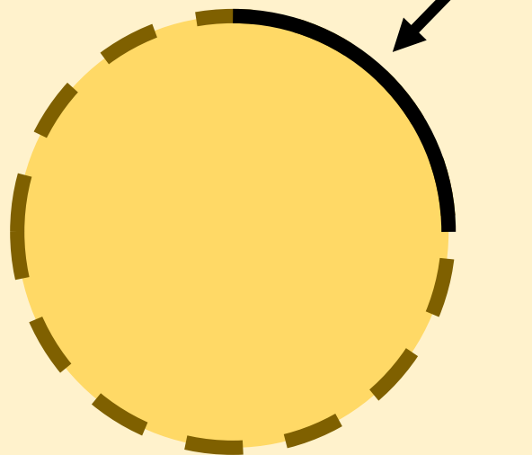
Arc
